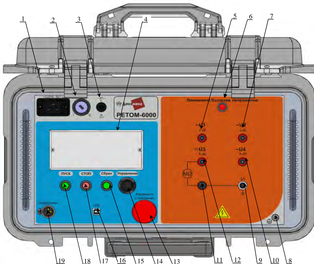
Рисунок 2 – Лицевая панель РЕТОМ-6000
